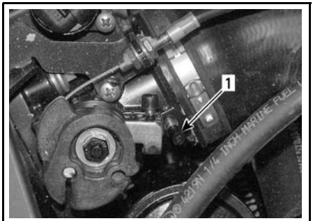
lmo2007-001-008_a REMOVE CAP 1. Plastic cap
