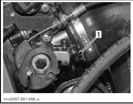
REMOVE CAP 1. Plastic cap
