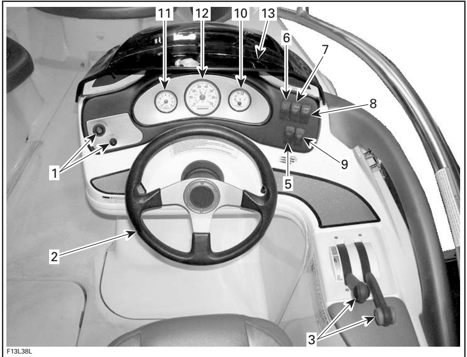
TYPIQUE — VUE DU POSTE DE PILOTAGE
