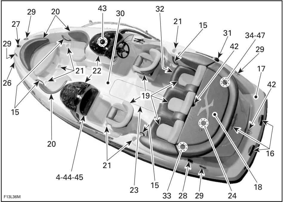
TYPIQUE — VUE SUPÉRIEURE
