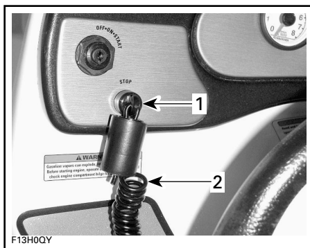
TYPIQUE — INTERRUPTEUR D'ARRÊT ET CORDON DE SÉCURITÉ
