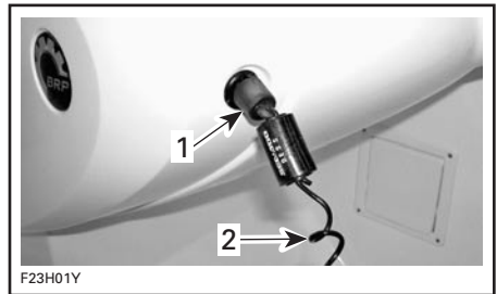
TIPIQUE — INTERRUPTEUR D'ARRÊT ET CORDON DE SÉCURITÉ
