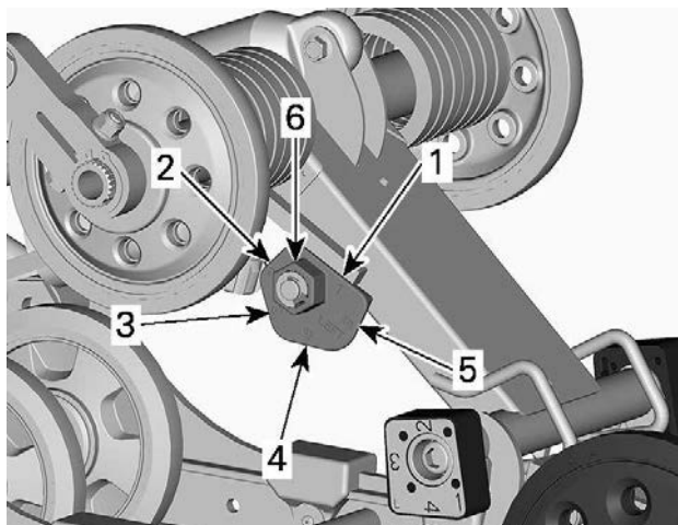
RMOTION，不带快速调节系统 - 左侧
