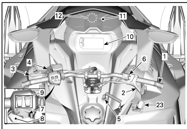
600R E-TEC-MOTOR
