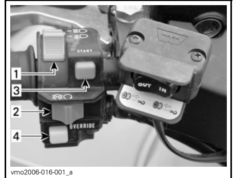
TÍPICO—INTERRUPTOR MULTIFUNÇÕES
