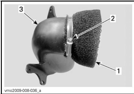
ENTRADA DE AR DA CVT RETIRADA PARA UMA MAIOR CLAREZA
