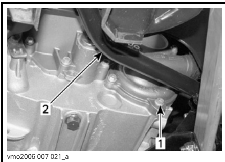
1. Tampão de drenagem do líquido de arrefecimento 2. Pedal do travão
