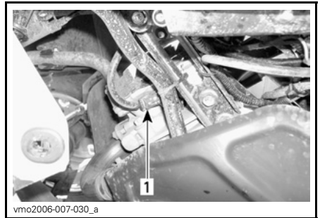
CILINDRO FRONTAL — DO LADO ESQUERDO 1. Vela de ignição
