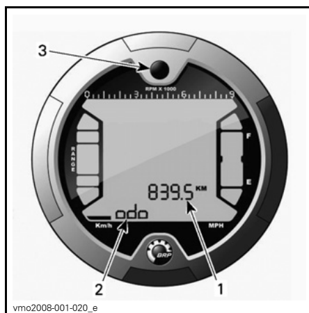
1. Visor 2 (modo) 2. Visor 3 (modo/mensagem) 3. Botão do selector
