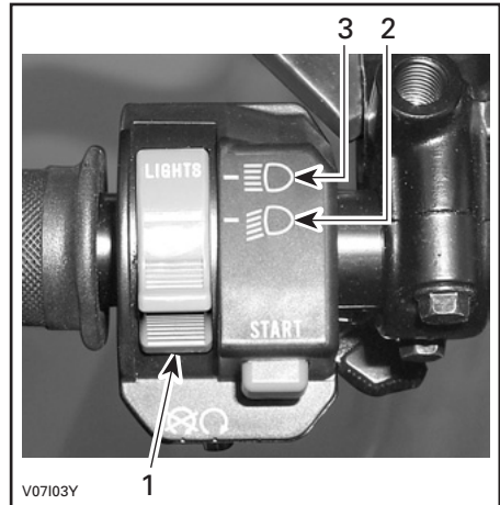
FUNÇÕES DO INTERRUPTOR DO FAROL DA FRENTE
