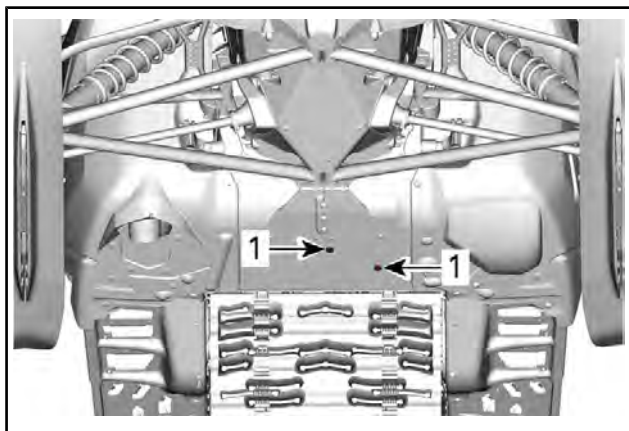
1. Trappe d'accès aux bouchons de vidange
