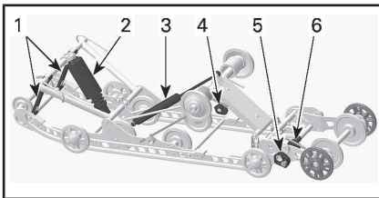
SC5-U 后悬架
