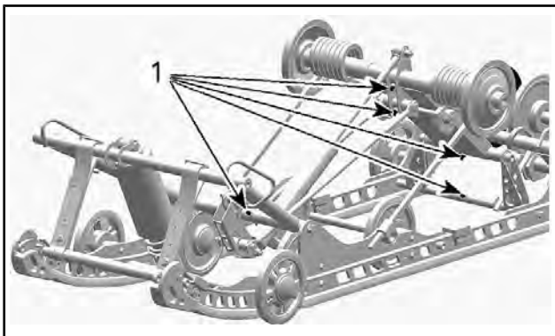
1. Smörjnipplar
