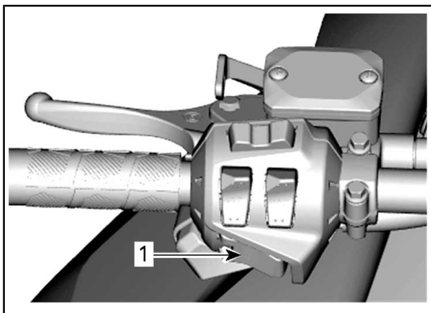
1. Taste Start / RER (elektromechanisch)
