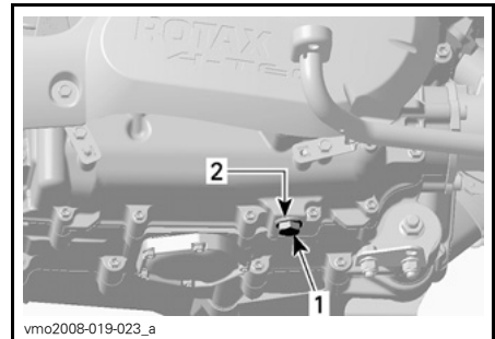
RECHTERKANT VAN DE MOTOR 1. Olieaftapplug 2. Pakkingring
