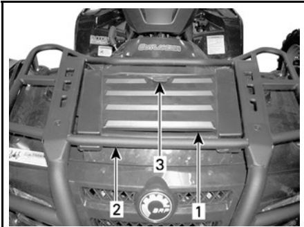
vmo2006-005-026_a 1. Paneel servicecompartment vooraan 2. Voorrek 3. Grendel
