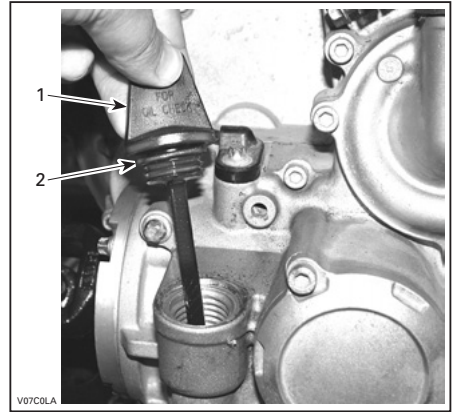
RECHTERKANT VAN DE MOTOR 1. Peilstok 2. O-ring
