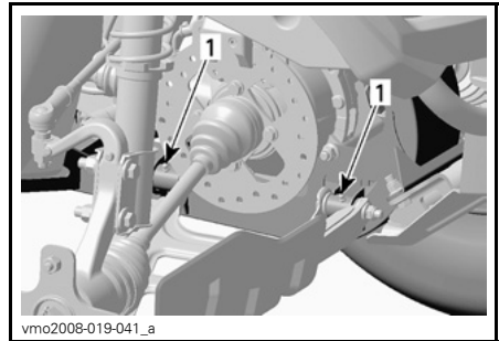
TYPISCH — RECHTS 1. Smerefittingen
