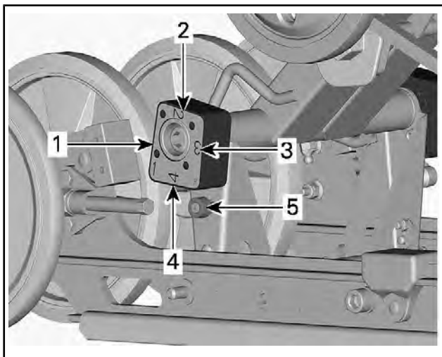
联接块 - 右侧视图
