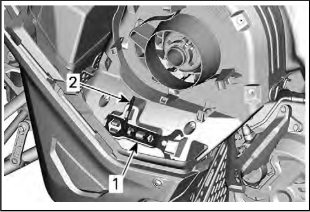
典型示例 - 驱动皮带护罩工具位置
