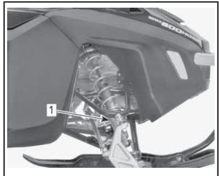
代表例 - カムタイプのプリロード
