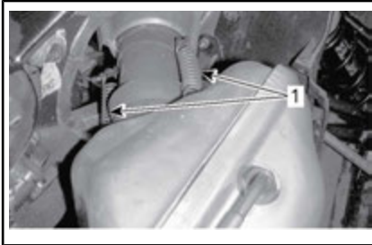
TYPBILD - 600 HO E-TEC (FRÅN FORDONETS HÖGRA SIDA)
