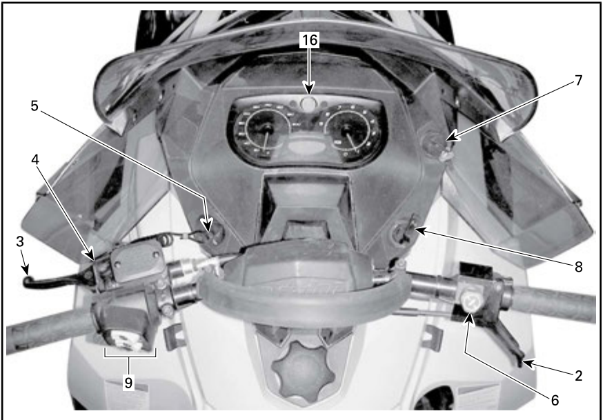
TYPBILD - 550F-MODELLER
