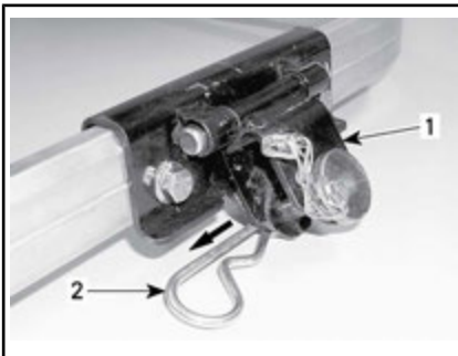
TILHENGERFESTE (C-TYPE)
