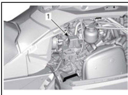
1. Sikringsboks
