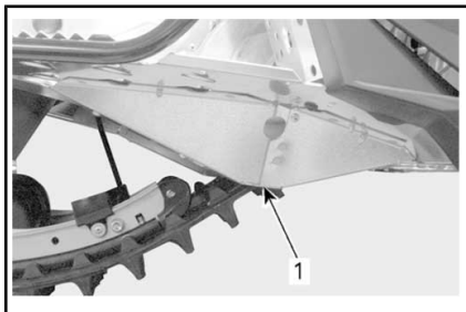
1. Dräneringspluggens åtkomsthål
