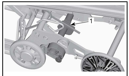
1. Förspänningskam
