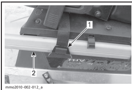
1. Удерживающий ремень 2. Задний бампер
