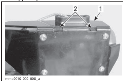
1. Монтажная пластина 2. Прорезы
