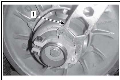
调节器轮毂
