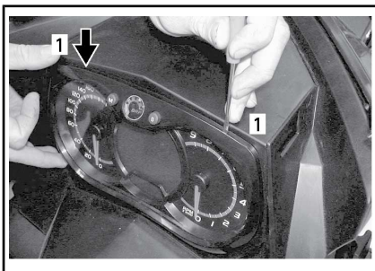
1. 锁定片
