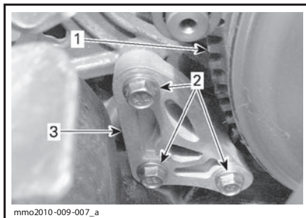
1. Ведущий шкив вариатора 2. Винты крепления упора двигателя 3. Упор двигателя
