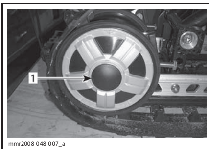
1. Колпак правого заднего натяжного катка
