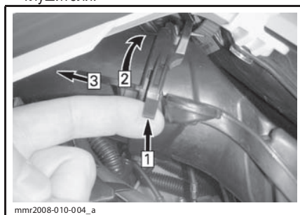
ТИПОВОЙ ВАРИАНТ Шаг 1: Поднять фиксатор Шаг 2: Повернуть адаптер Шаг 3: Сдвинуть
