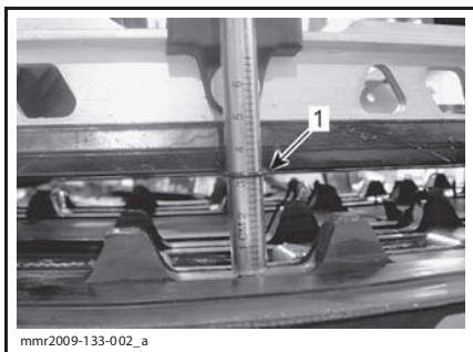
1. Нижнее кольцо вровень с нижней кромкой наклейки полоза
