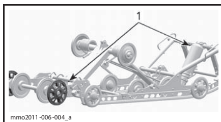
1. Пресс-масленки
