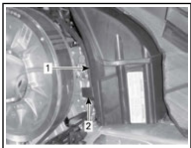
1. Silencieux d'admission d'air primaire 2. Languette de verrouillage du silencieux d'admission primaire
