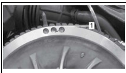
典型示例 - 初步设置
