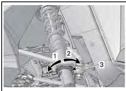
凸轮类型 - 运动控制减震器
