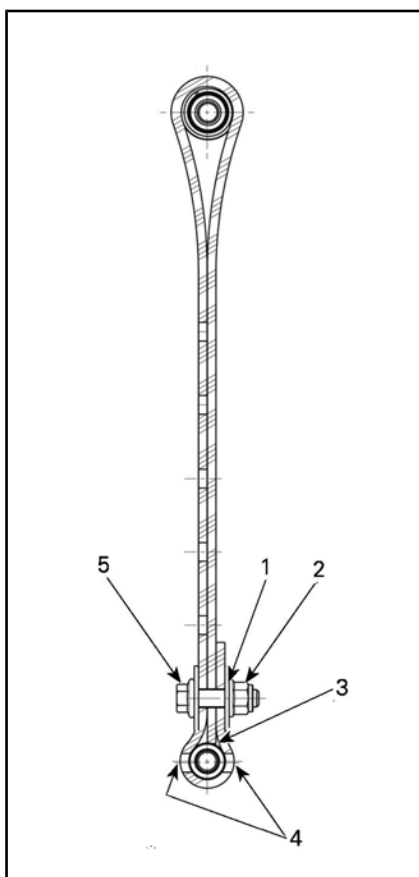
止动带位置 1 (第 1 个孔, 最长)
