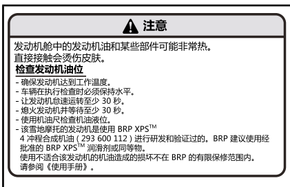
1200 4-TEC 型 - 位于发动机舱内
