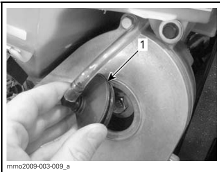
TYYPILLINEN - KETJUKOTELON YLÄOSA 1. Täyttökorkki
