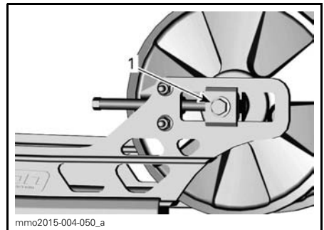
tMOTION 1. Boulon de roue de support arrière gauche
