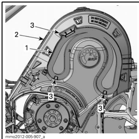
1. Courroie d'entraînement de rechange 2. Garde-courroie d'entraînement 3. Languettes de fixation
