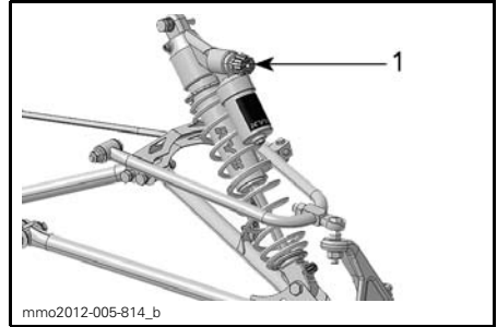
1. Dispositif de réglage de force de compression
