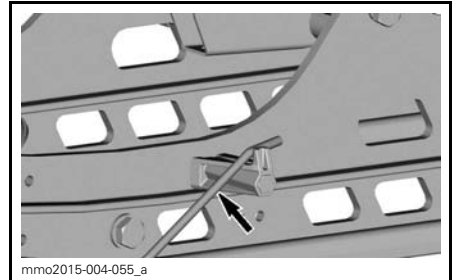
GRATTOIRS À NEIGE EN POSITION RABATTUE
