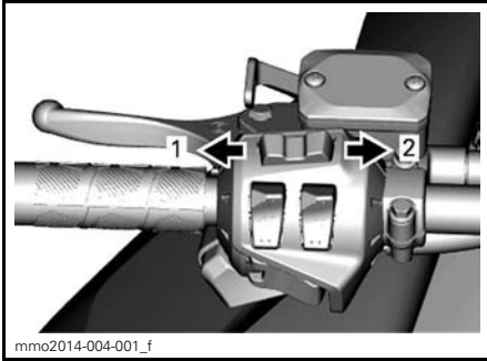
COMBINÉ D'INTERRUPTEURS
