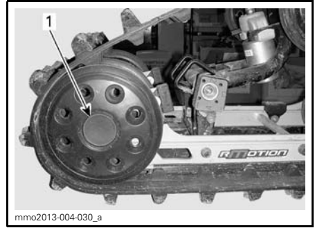
rMOTION 1. Enjoliveur de roue arrière droite
