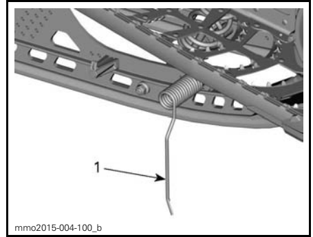
TYPIQUE - CERTAINES PIÈCES ONT ÉTÉ RETIRÉES À DES FINS DE CLARTÉ 1. Grattoir à neige en position active
