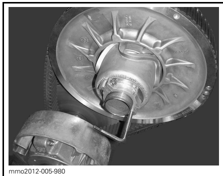
MANDRIN DE POULIE MENÉE INSTALLÉ SUR LE DISPOSITIF DE RÉGLAGE
