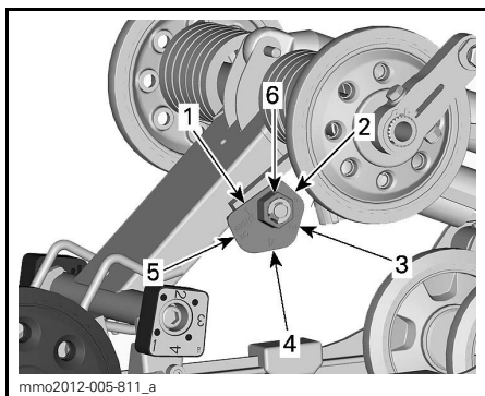
rMOTION SANS BOUTON DE RÉGLAGE RAPIDE - CÔTÉ DROIT
