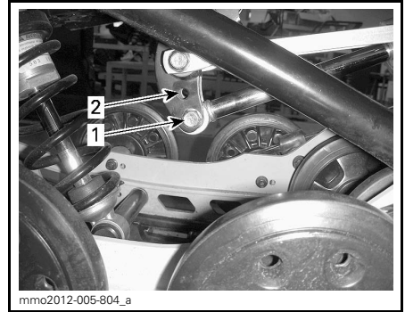
POSITION DE FIXATION DE L'AMORTISSEUR ARRIÈRE 1. Position haute performance 2. Position sport
