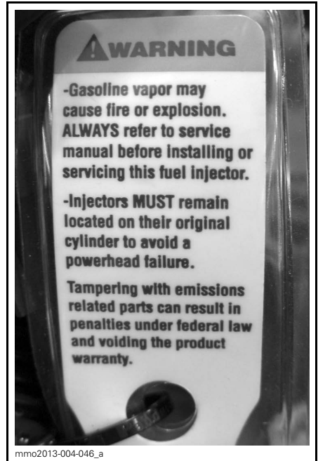
ÉTIQUETTE 15 - SUR LES INJECTEURS
