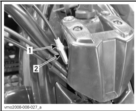
1. Contratuerca 2. Ajustador
