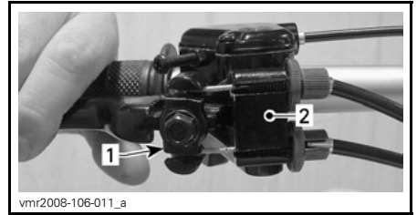
1. Conexión para cables 2. Soporte para cables
