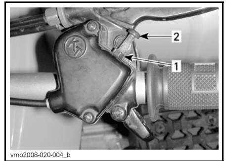
1. Contratuerca 2. Tornillo limitador de velocidad
