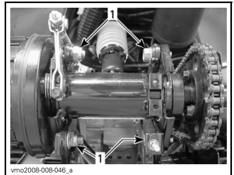
TÍPICO — EJE TRASERO 1. Pernos de bloqueo
