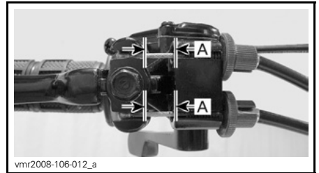
A. 10 y 12 mm (13/32 de pulgada y 1/2 pulgada)
