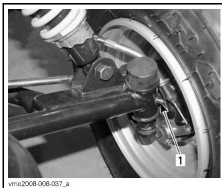
TÍPICO 1. Engrasador
