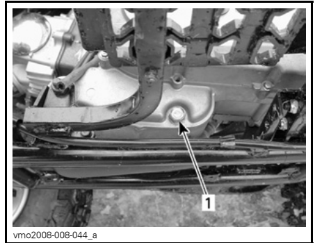
PARTE IZQUIERDA DEL MOTOR 1. Tapón de drenaje
