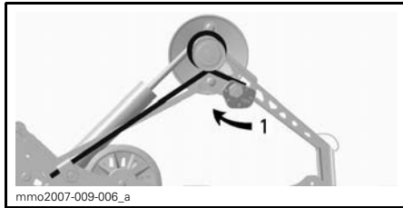
TIPIQUE — CÔTÉ GAUCHE 1. Régler la précharge du ressort
