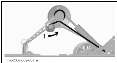
TIPIQUE — CÔTÉ DROIT 1. Régler la précharge du ressort
