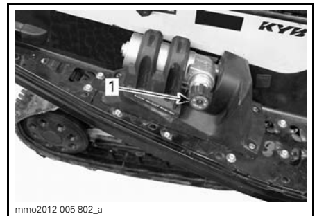
1. Bouton pour régler la compression à basse ou à haute vitesse
