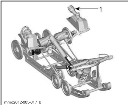
rMOTION À BOUTON À RÉGLAGE RAPIDE 1. Bouton de gauche pour régler la précharge
