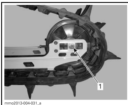
1. Vis de fixation de roue de support arrière gauche
