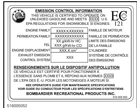
ÉTIQUETTE DE CONFORMITÉ 1 - DANS LE COMPARTIMENT MOTEUR
