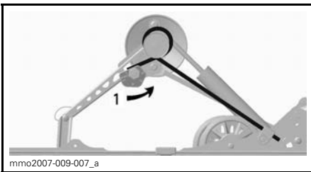
TIPIQUE — SC-5 — CÔTÉ DROIT 1. Régler la précharge du ressort
