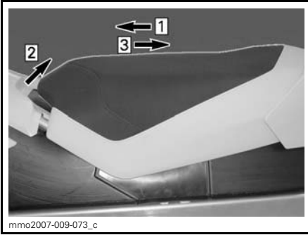
SIÈGE INSTALLÉ
