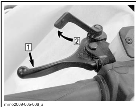
TYPIQUE — POUR VERROUILLER LE MÉCANISME
