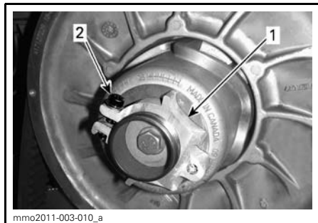
1. Anneau de réglage 2. Boulon de serrage
