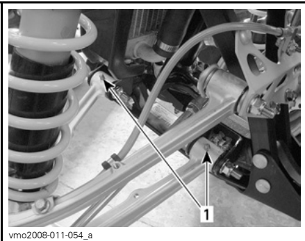
TYPBILD — UNDRE BÄRARM 1. Smörjnippel
