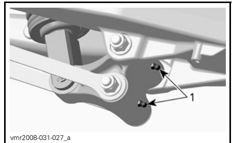
VINKELHÄVARM 1. Smörjnippel
