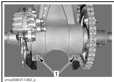
1. Bakaxelns låsbultar
