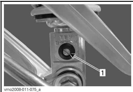
ALLA MODELLER 1. Returdämpningsjusterare (flat skruvmejsel)
