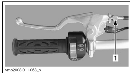
1. Vajerjusterare
