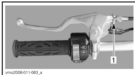
1. Låsmutter
