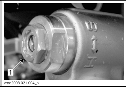
TYPBILD — ENDAST X XC-PAKET 1. Kompressionsjusterare, hög hastighet (17 mm-nyckel)
