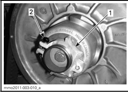
1. Dispositif de réglage 2. Vis de serrage
