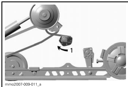
TIPIQUE — CÔTÉ GAUCHE 1. Régler la précharge du ressort
