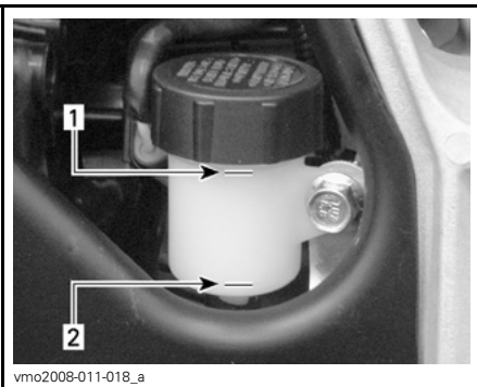
HØYRE SIDE AV ATVEN 1. Maksimumsnivå (MAX) 2. Minimumsnivå (MIN)
