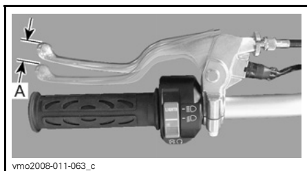
CLUTCHHÅNDTAK NORMAL DØDGANG A. 10 til 15 mm (3/8 til 5/8 tommer)
