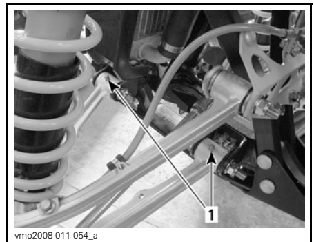
TYPEBILDE NEDRE OPPHENGSAARM
