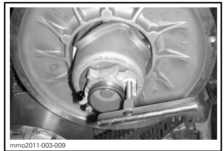
MANDRIN DE POULIE MENÉE SUR UN DISPOSITIF DE RÉGLAGE EN ALUMINIUM
