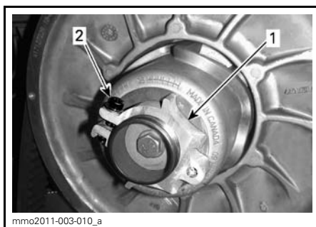
mmo2011-003-010_a DISPOSITIF DE RÉGLAGE EN ALUMINIUM
