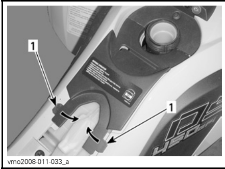
1. Linguette
