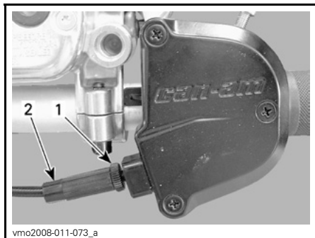
1. Controdado 2. Registro
