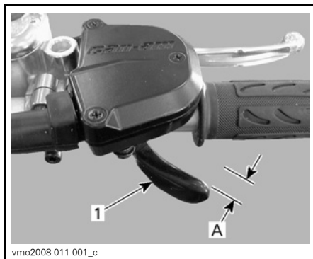
1. Leva dell'acceleratore
