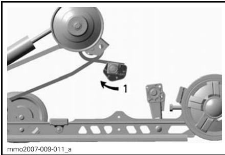
TIPIQUE — SC-5 — CÔTÉ GAUCHE 1. Régler la précharge du ressort
