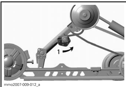
TIPIQUE — SC-5 — CÔTÉ DROIT 1. Régler la précharge du ressort
