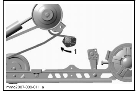
TYPBILD — VÄNSTER SIDA 1. Justera fjäderförspänningen
