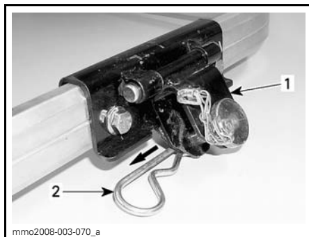
1. Dragkrok 2. Låssprint
