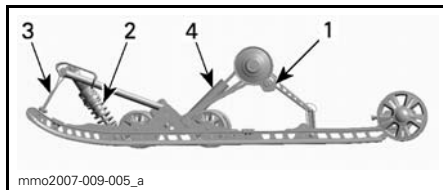
SC-5M™ BAKFJÄDRING (TUNDRA OCH TUNDRA SPORT)
