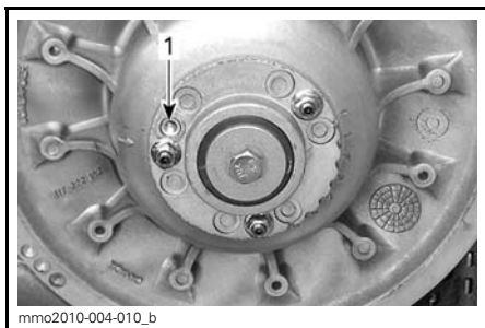
1. Gängat hål
