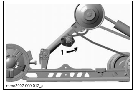
TYPBILD — HÖGER SIDA 1. Justera fjäderförspänningen
