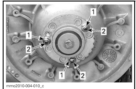
1. Låsemuttere 2. Justeringssskruer
