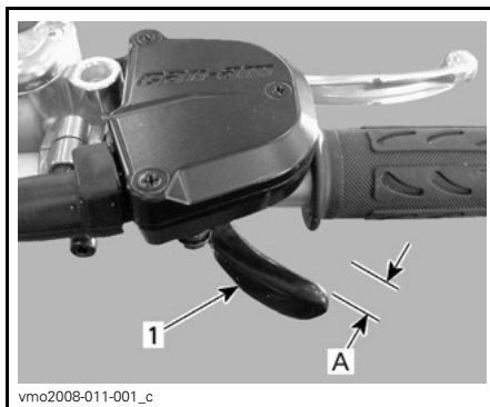
1. Palanca del acelerador A. 2 a 4 mm (5/64 a 5/32 de pulg.)
