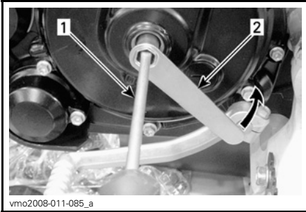
1. Destornillador 2. Llave de ajuste del embrague
