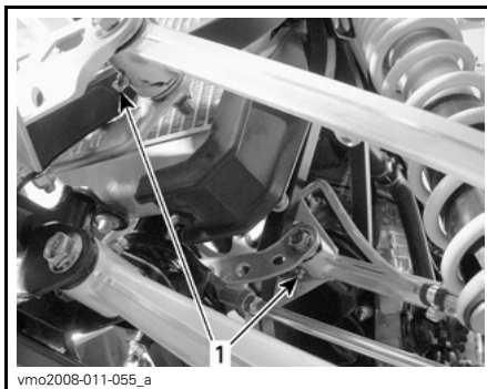
TÍPICO — BRAZO DE SUSPENSIÓN DE LA PARTE SUPERIOR (DS 450/DS 450 X XC)
