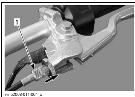
1. Ajustador del cable
