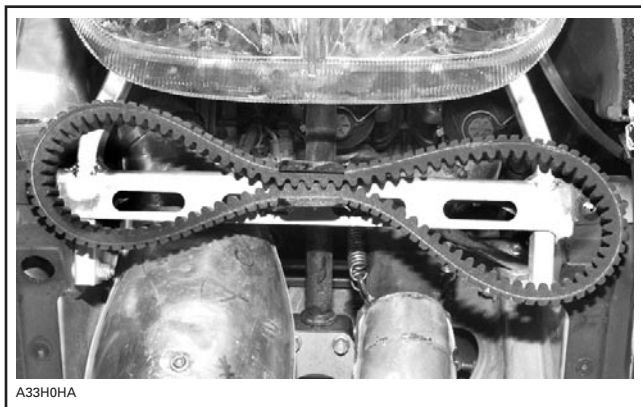
TYPIQUE — COURROIE DE RECHANGE EN PLACE DANS LE SUPPORT
