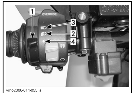
TYPEBILDE – FRONTLYSBRYTERENS FUNKSJONER
