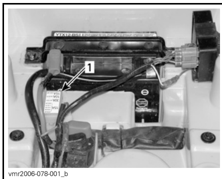
1. Sikringsholder
