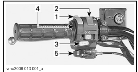
TYPEBILDE – FLERFUNKSJONSBRYTER
