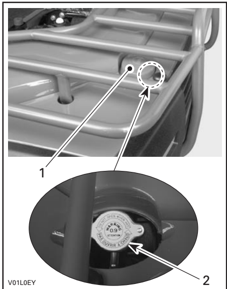
1. Capuchon protecteur 2. Bouchon de radiateur
