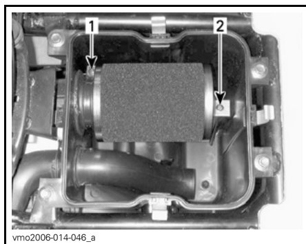
1. Klämman 2. Hållskruv
