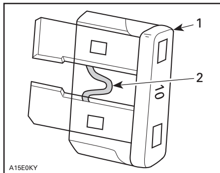
1. Säkring 2. Kontrollera om säkringen smält
