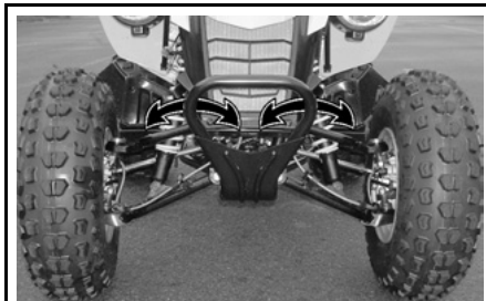
TYPBILD – PLACERING AV FRÄMRE STÖTFÅNGARREMMAR
