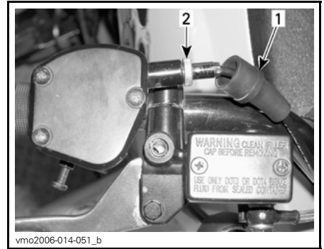
1. Rubberbeschermering 2. Kabelstelschroef
