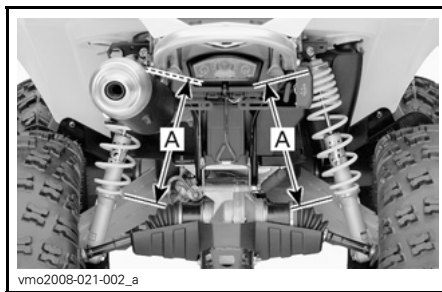
TÍPICO — AJUSTE PRÉ-CARGA — TRASEIRO A. Mesmo comprimento
