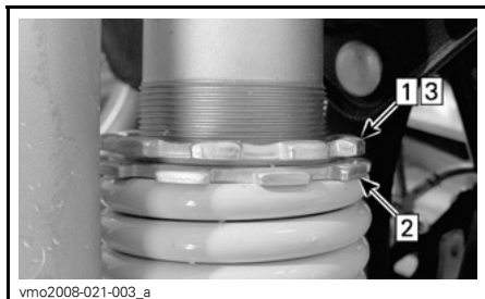
TÍPICO — AJUSTE PRÉ-CARGA — FRENTE A. Mesmo comprimento
