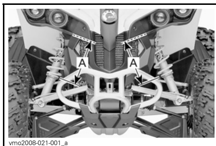
TÍPICO — AJUSTE PRÉ-CARGA — FRENTE A. Mesmo comprimento
