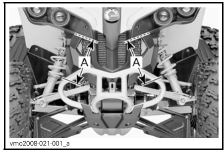
TYPISCH — REGELING VOORBELASTING — VOORAAN A. Zelfde lengte
