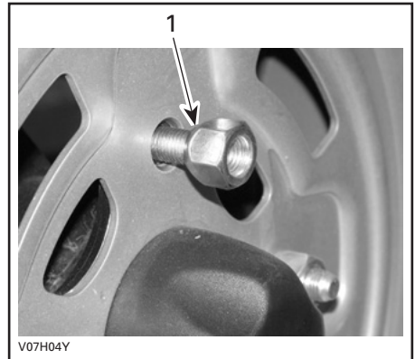
TYPISCH — TYP MIT OFFENEM ENDE 1. Konische Seite der Mutter
