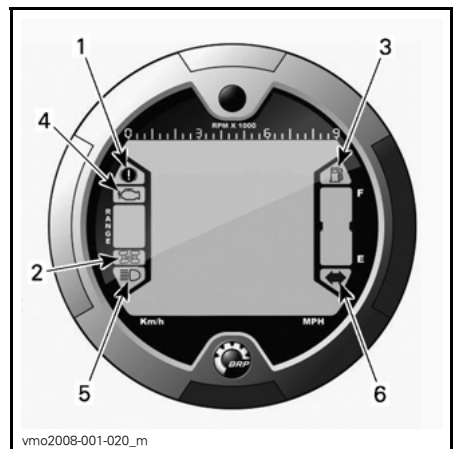
1. Anzeigeleuchte Standbremse 2. Anzeigeleuchte Allradantrieb 3. Anzeigeleuchte "Niedriger Kraftstoffstand" 4. Anzeigeleuchte motorüberprüfung 5. Fernlichtanzeigeleuchte 6. Blinkende Warnlampe
