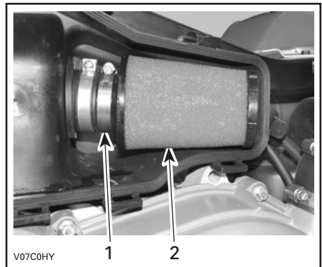
1. Fascetta 2. Filtro aria
