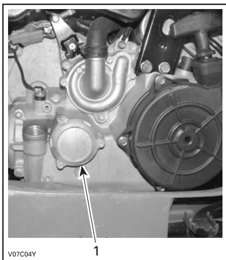
SITUAZIONE TIPICA 1. Coperchio filtro dell'olio
