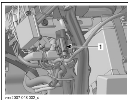
TIPICA — POSIZIONE FUSIBILE POSTERIORE 1. Alimentazione (30 A)
