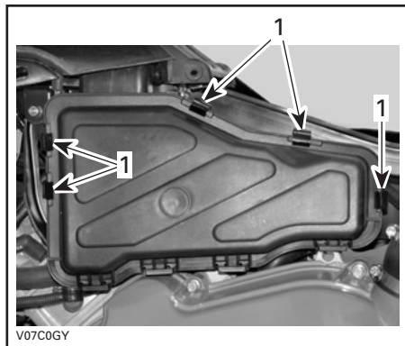
1. Sganciare fascette
