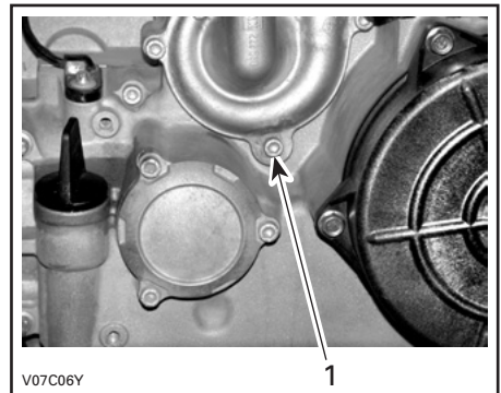
1. Tapón de drenaje de refrigerante
